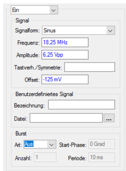
Einstellungen Kurvenformgenerator
