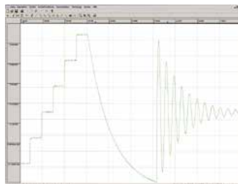
Kurvenformeditor des Funktions- und Arbitrarygenerators
